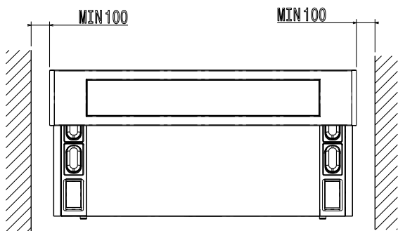
Felülnézet
